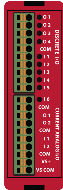
EZRPL-IO-6DI4DO-2ANI2ANOC
